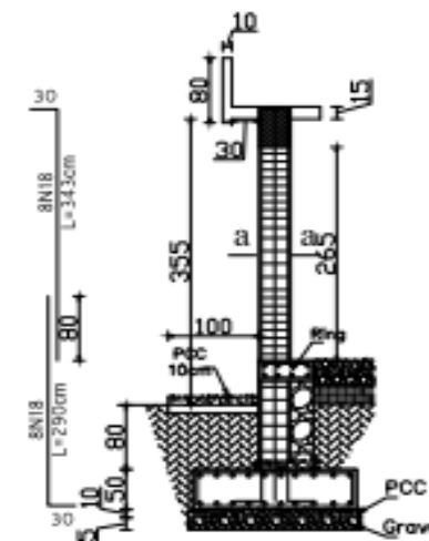
Sec(e-e)
