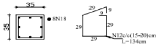
Sec(a-a)
